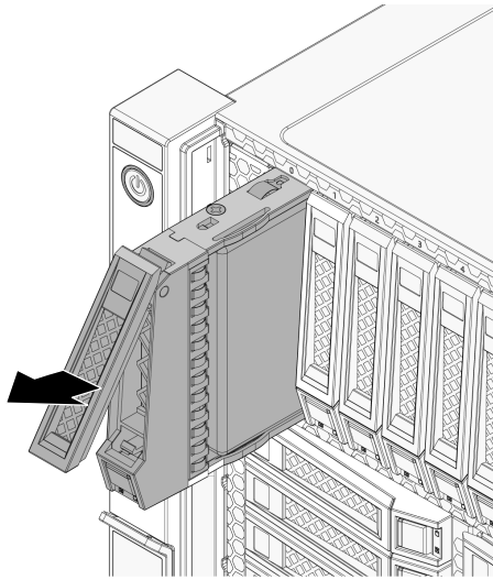
图 4-29 拉出硬盘模组
