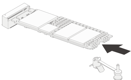
图 4-11 安装 M.2 硬盘
