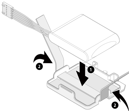
图 4-7 安装超级电容
