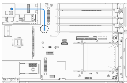
图 4-3 入侵开关接口位置
