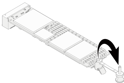
图 4-9 拆除 M.2 硬盘固定卡扣
