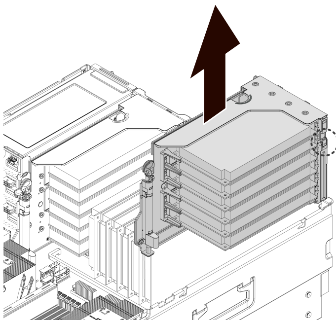
图 4-25 拆卸 PCIe Riser 卡模组
