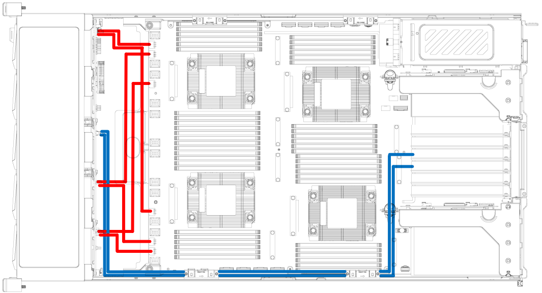
图 4-36 50 × 2.5 英寸 SATA/SAS+18PCIe 配置
