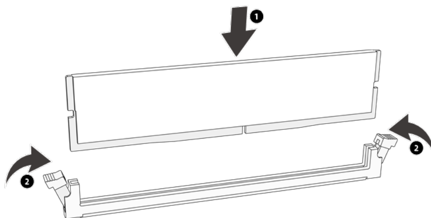
图 4-16 安装内存示意图
