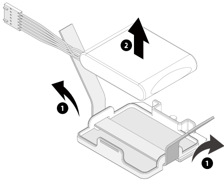
图 4-6 拆除超级电容
