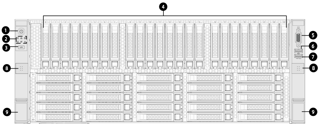
图 3-1 49 × 2.5 英寸盘位前窗示意图
