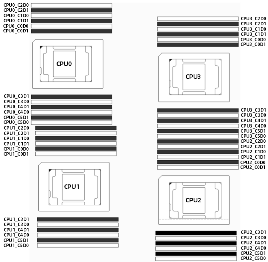
图 4-17 内存插槽布局
