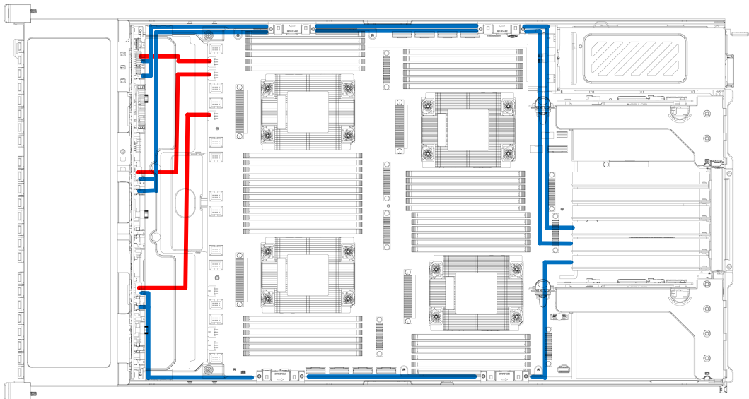
图 4-34 24 × 2.5 英寸 SATA/SAS+18PCIe 配置
