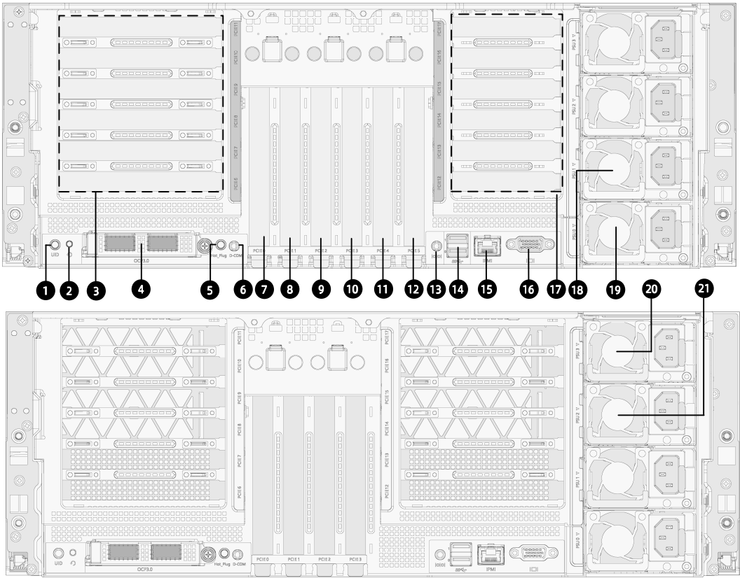
图 3-3 后面板示意图
