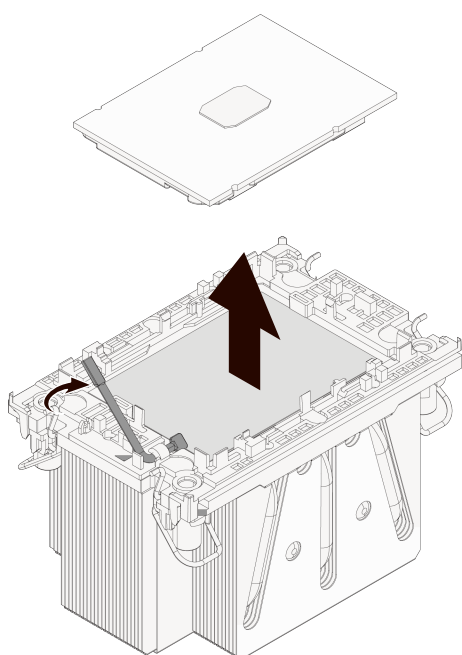
图 4-19 拆卸 CPU
