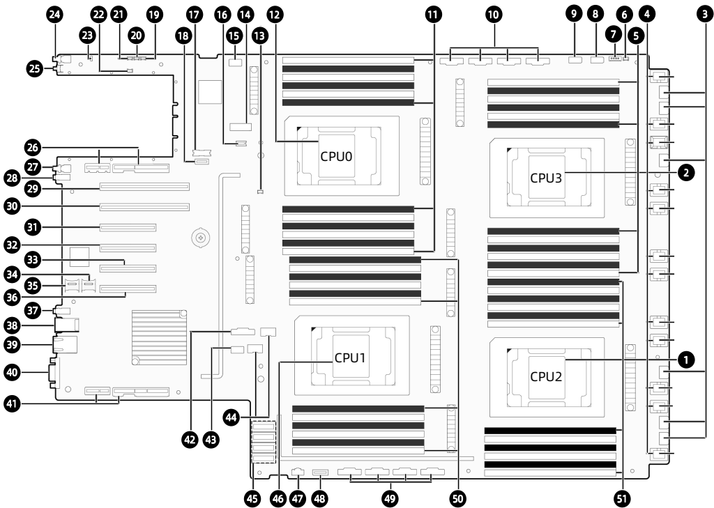
图 3-5 主板示意图
