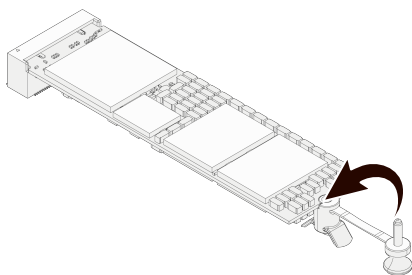
图 4-12 安装 M.2 硬盘固定卡扣
