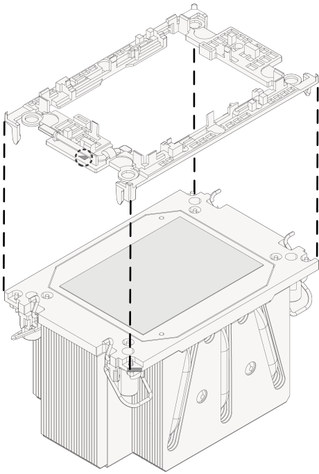
图 4-20 拆卸 CPU 固定架
