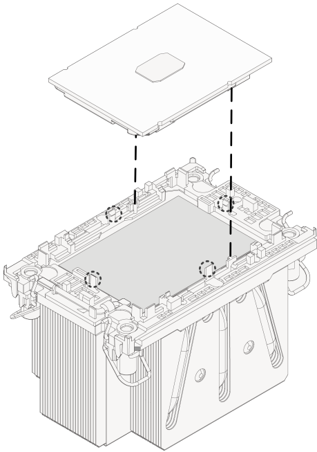
图 4-22 安装 CPU
