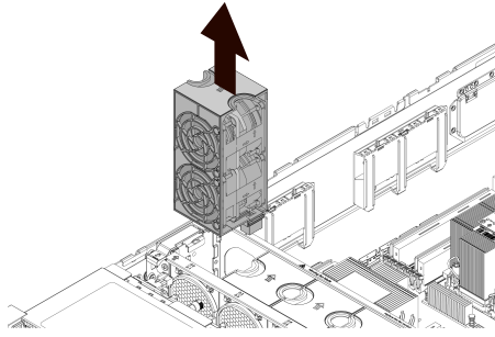
图 4-23 拆卸风扇模组
