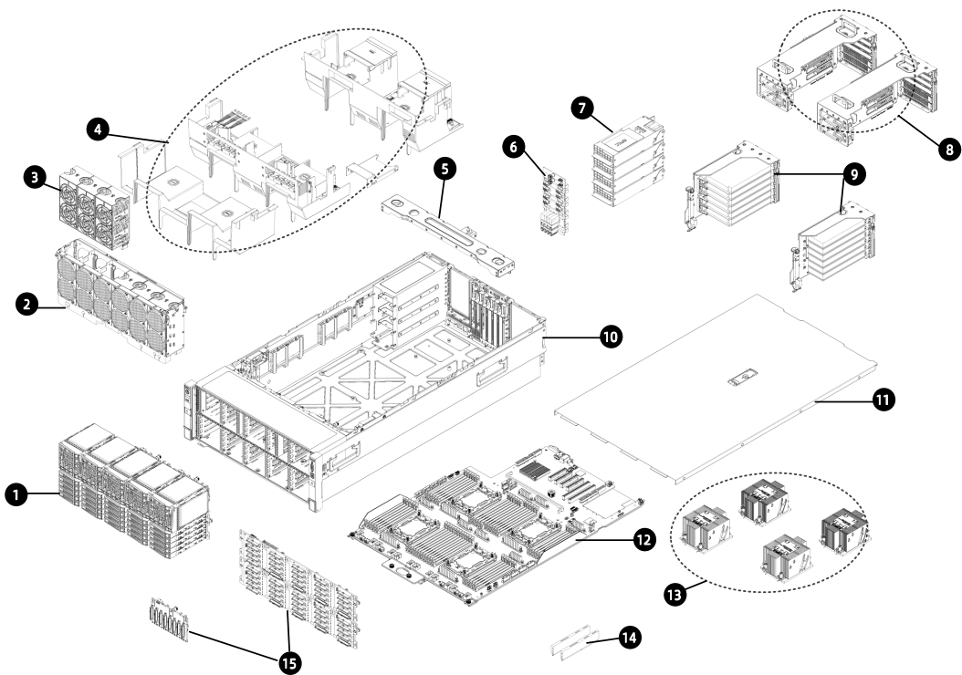
图 3-6 爆炸图
