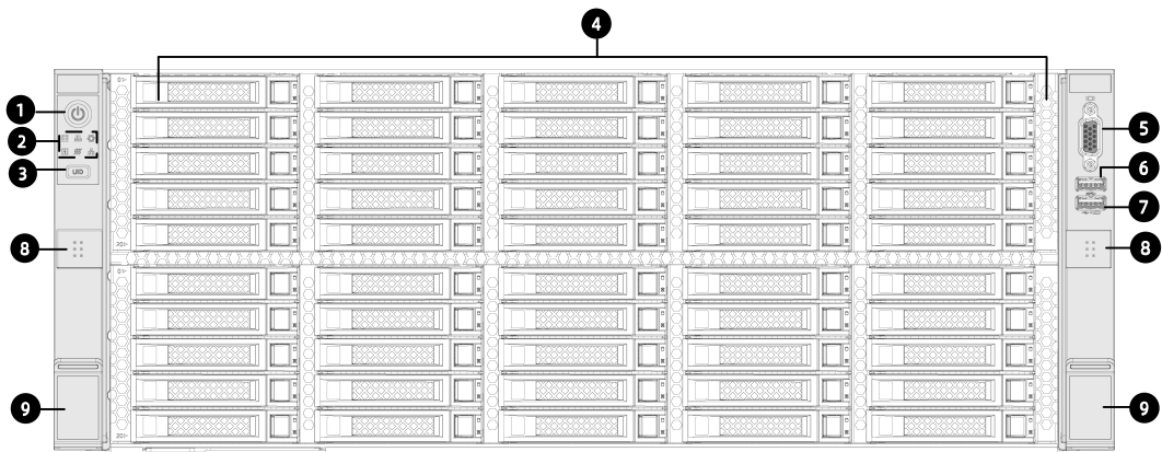
图 3-2 50 × 2.5 英寸盘位前窗示意图
