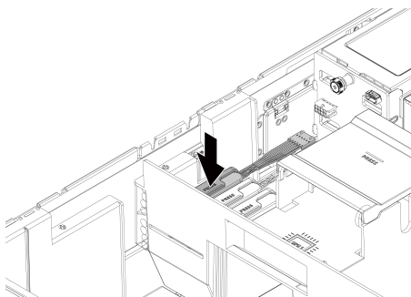
图 4-4 按压超级电容支架顶部
