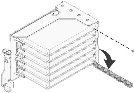
图 4-26 打开 PCIe 盖板
