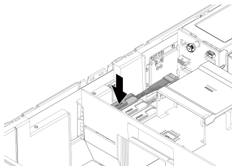
图 4-8 安装超级电容到导风罩
