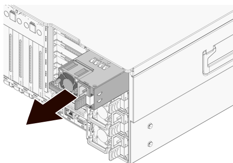
图 4-31 拆卸电源
