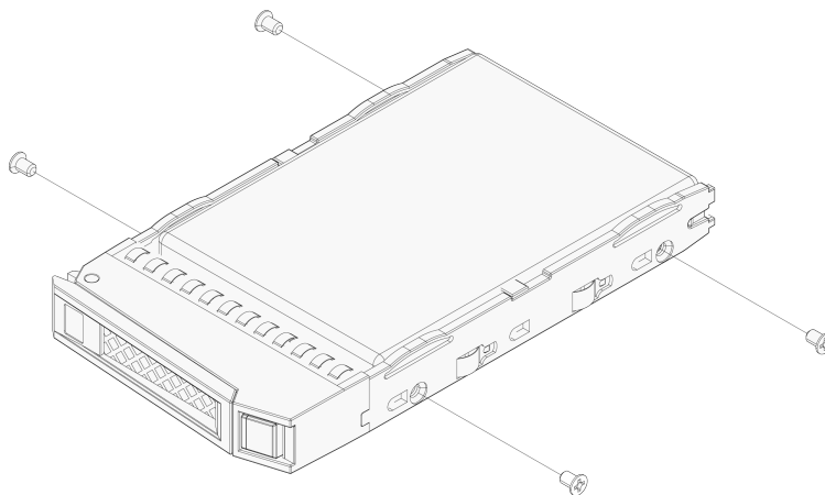
图 4-30 拆卸硬盘固定螺丝示意图
