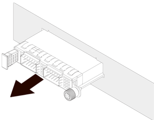
图 4-33 抽出 OCP 卡
