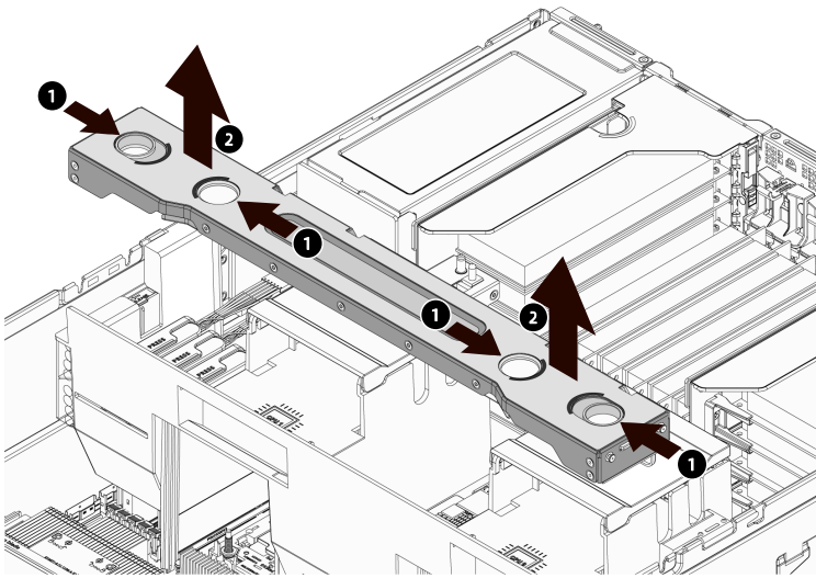
图 4-13 拆下中支架
