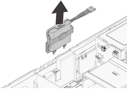
图 4-5 取出超级电容支架
