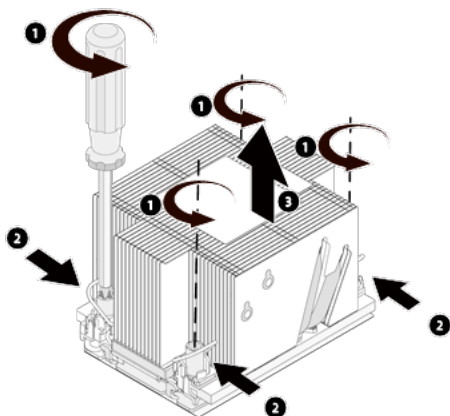
图 4-18 拆卸 PHM
