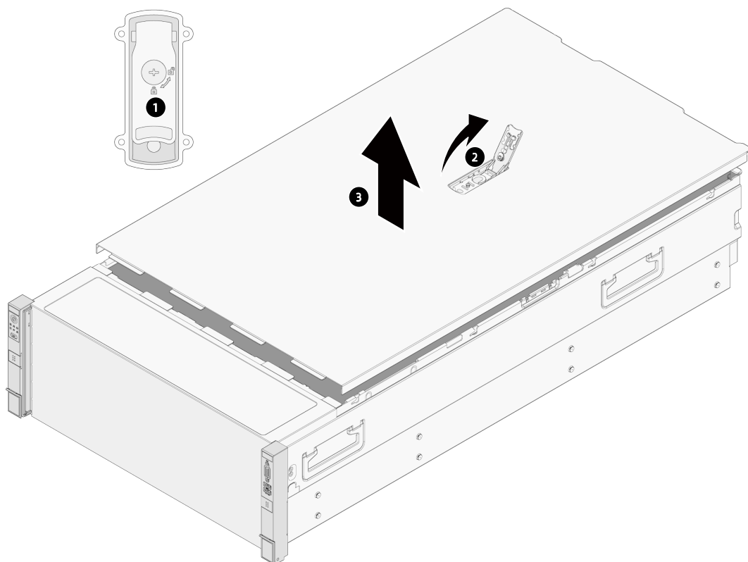
图 4-2 拆卸机箱上盖
