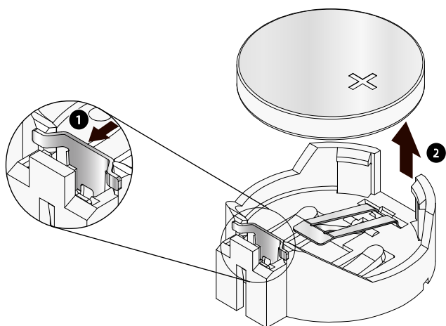
图 5-1 取出电池
