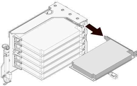
图 4-27 拔出 PCIe 卡
