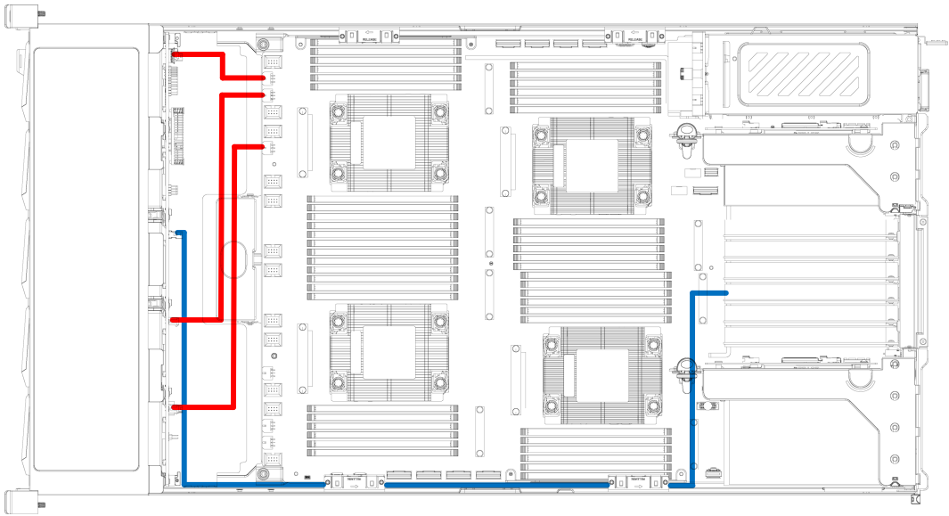
图 4-35 25 × 2.5 英寸 SATA/SAS+18 PCIe 配置
