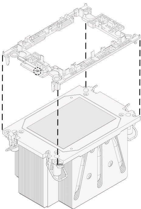
图 4-21 安装 CPU 固定架
